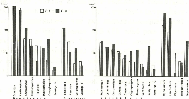
Abb.1: Schlüpfabundanz (bzw. Aktivitätsdichte) von Insektenimagines (1971) in Fichtenwäldern des Solling (F 1 ca. 90jährig; F 3 ca. 40jährig; - s.(1). Diptera und Coleoptera nach Fam. getrennt; Reihenfolge nach Abundanzhöhe in F 1 (9).
